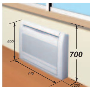
Sotto una finestra (unità: mm)
